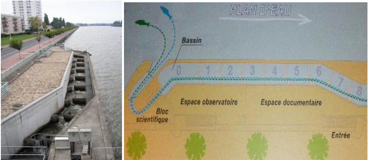
Figure 1 : Photographie et plan de la partie supérieure de la passe à poisson.
